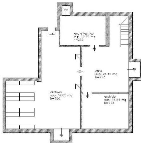
BRESCIA VIA D. VIOTTI 5 piano interrato
